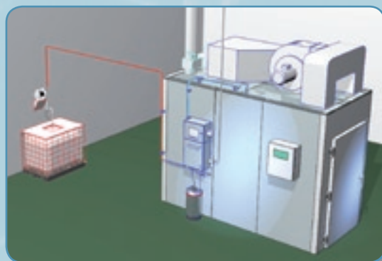
Når TARBER SMOKE MASTER monteres, behøves der ikke længere et lager med træflis eller kostbare luftrensesystem. En palle røgkondensat modsvarer 4-5 paller træflis.
